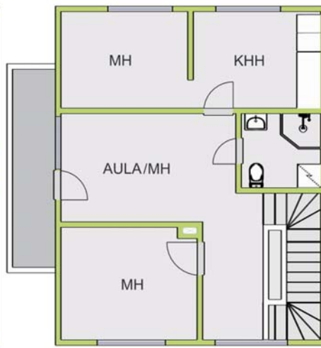
YLÄKERTA
