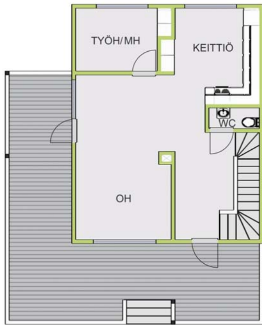
1. KERROS
